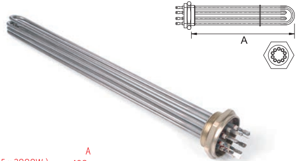
759 7500 W 300 mm. 760 10000 W 400 mm.
