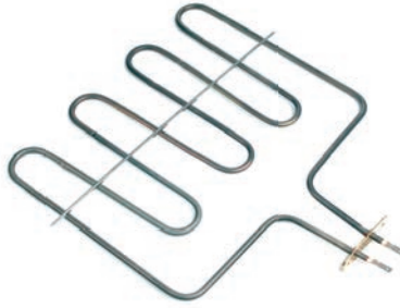
BR 14 Ø 6.5-8.5 mm Cr-Ni 230 V
