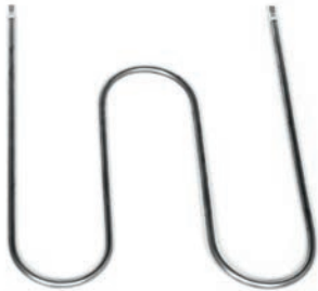
FM31 Ø 6.5-8.5 mm Cr-Ni 230 V 800W
