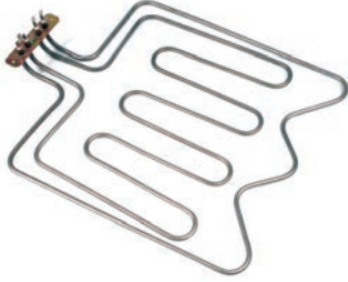
118 Ø 6.5-8.5 mm Cr-Ni 230 V 2000+1500W
